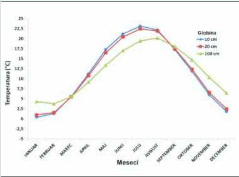
Povprečne mesečne temperature tal na različnih globinah za obdobje 1980–2014
