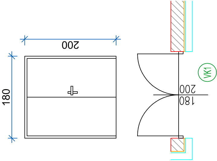
VK1 - 1 kom zunanja kovinska vrata; element vrat vel. 2x90 x 200 cm sistemska ključavnica vgradnja v opečno steno
