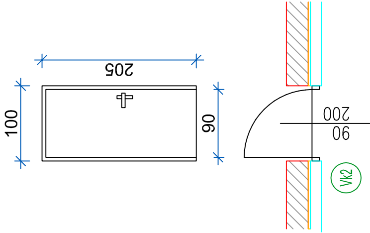
VK2 - 1 kom zunanja kovinska vrata; element vrat vel. 90 x 200 cm sistemska ključavnica vgradnja v opečno steno
