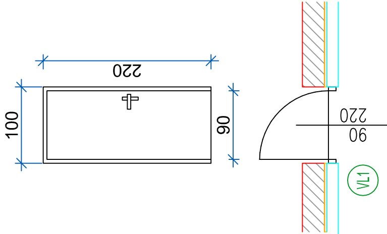
VL1 - 1 kom zunanja lesena vrata; element vrat vel. 90 x 220 cm podboj in krilo leseno, v beli barvi sistemska ključavnica samozapiralo vgradnja v opečno steno
