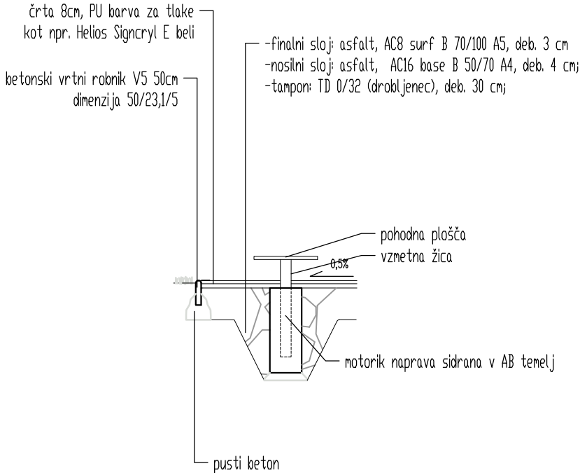
PREREZ
