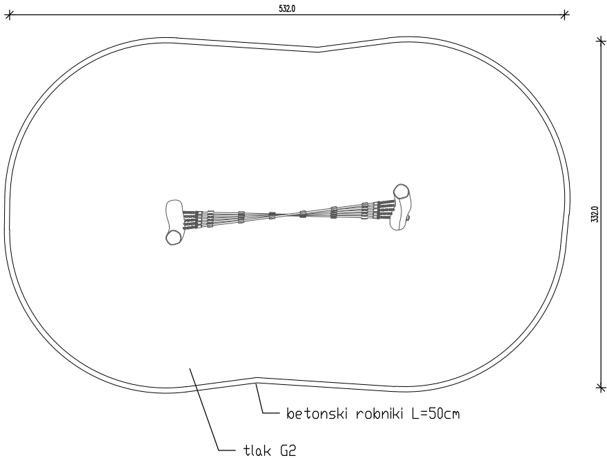
TLORIS
