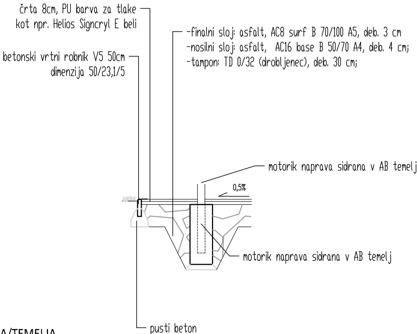
PREREZ TLAKA/TEMELJA
