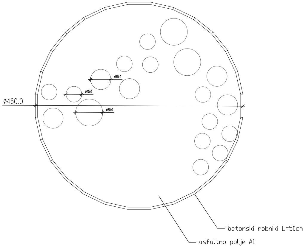
TLORIS
