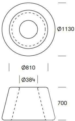
naslonjalo/korito
