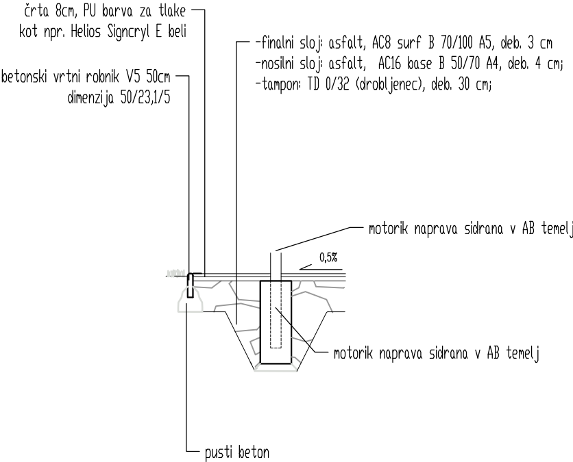
PREREZ TLAKA/TEMELJA
