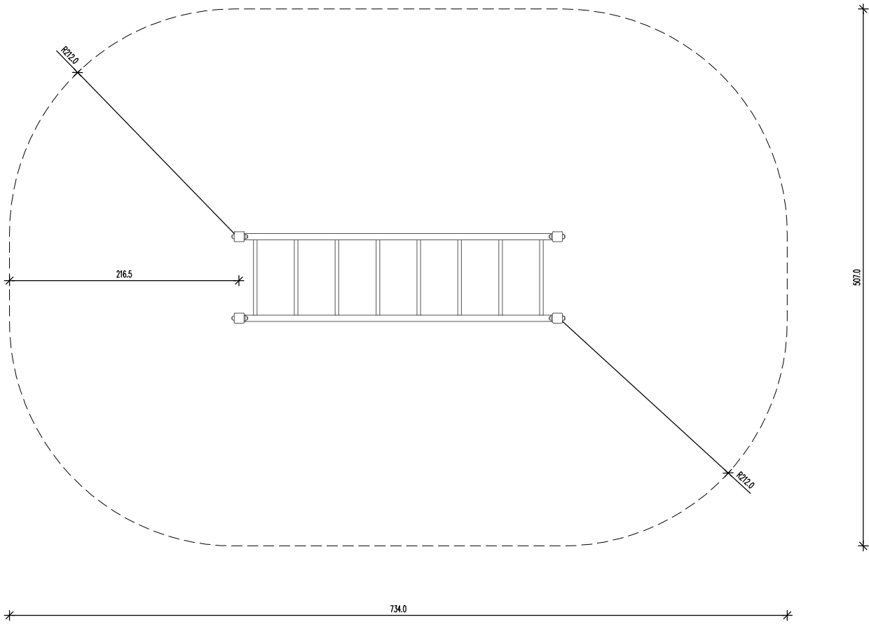
TLORIS
