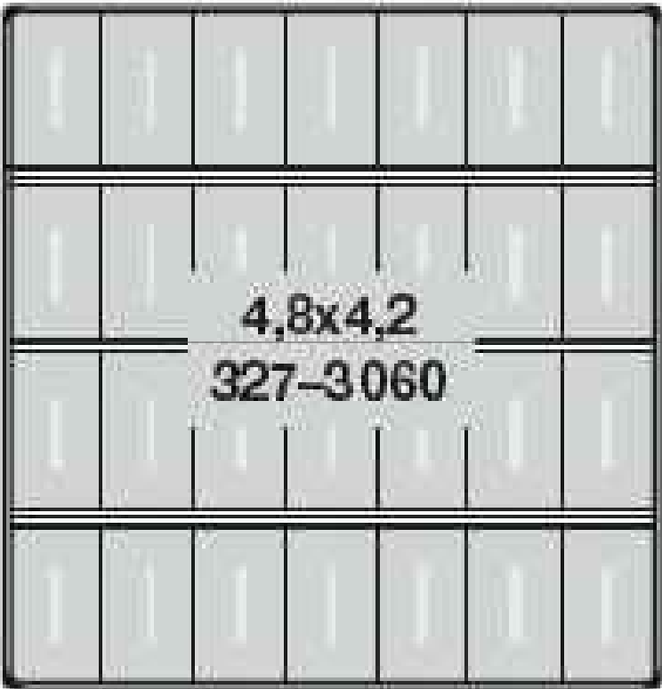
TLORIS PLOŠČADI 4,8X4,2m, nosilnost 3060kg
