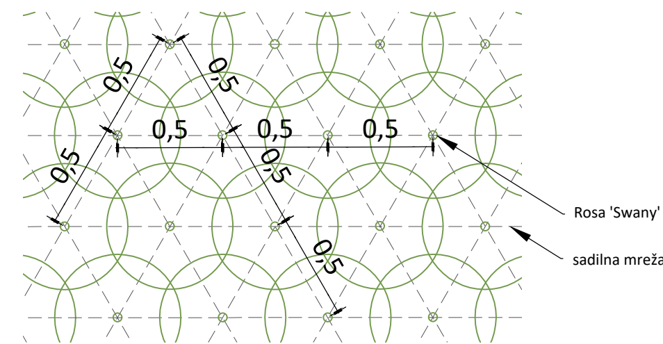
D1 - DETAIL SAJENJA POKROVNIH VRTNIC, M 1:25 - sadilna razdalja 0,5 m - cca. 4,5 km 2
