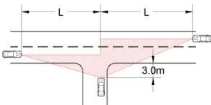
Slika 2: Primer varnostnega preglednostnega trikotnika (povzeto po Zakonu o cestah)
