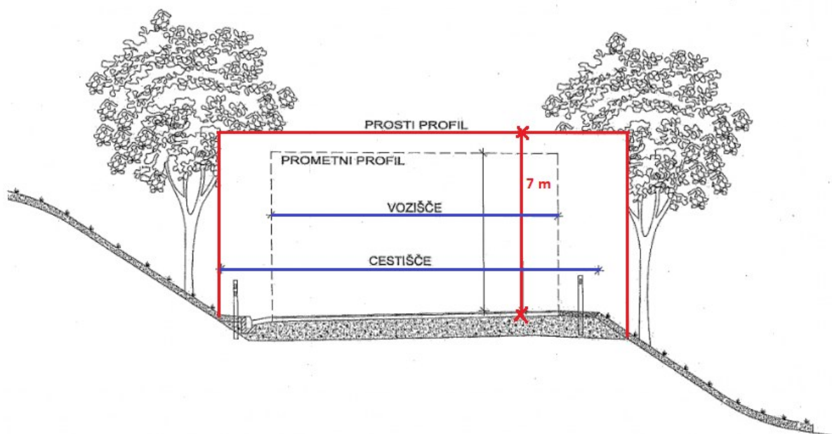
Slika 1: Zračni prostor nad cestiščem (povzeto po Zakonu o cestah)
