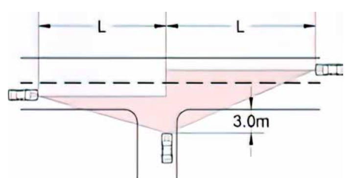
Primer varnostnega preglednostnega trikotnika (povzeto po zakonu o cestah).
