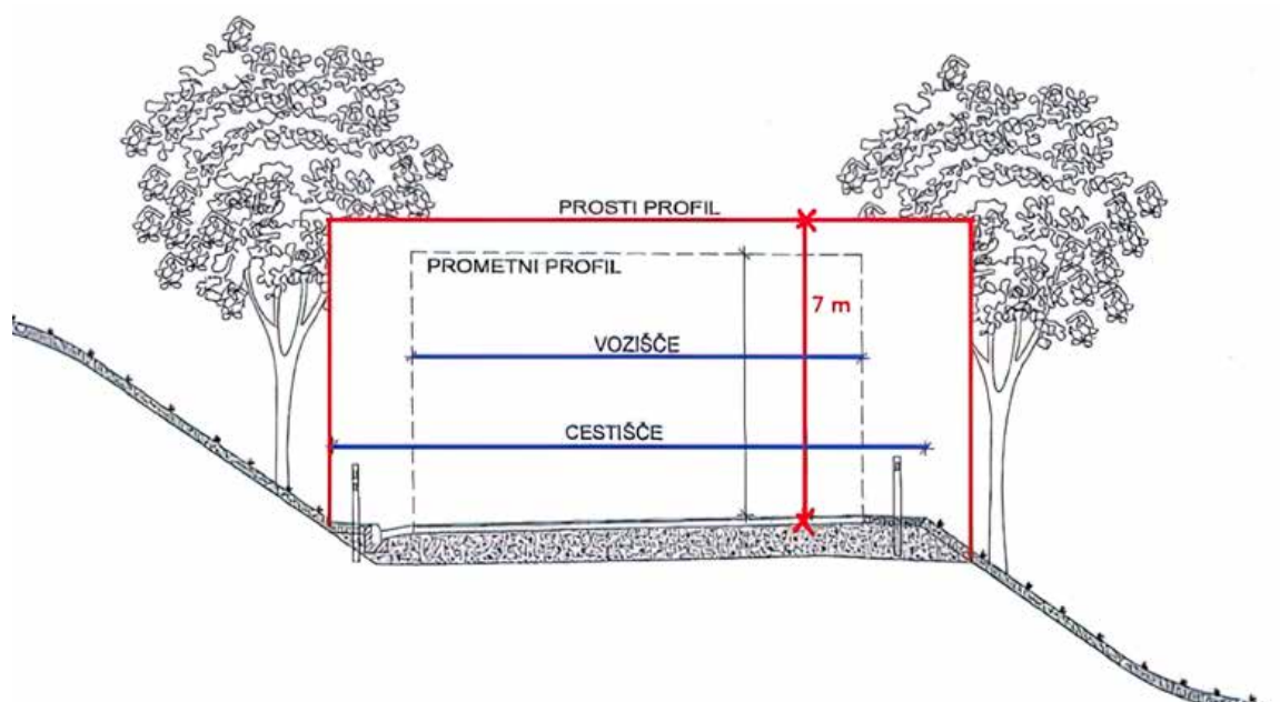
Zračni prostor nad cestiščem (povzeto po zakonu o cestah).
