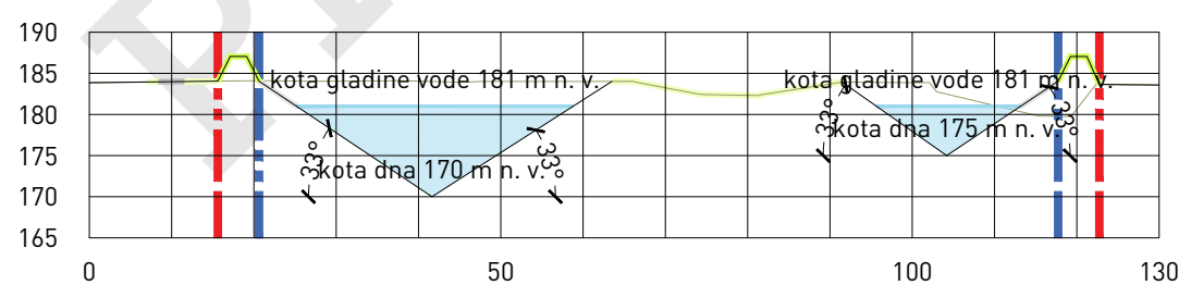
Profil D - D'
